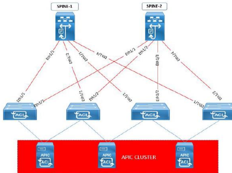
Figura 1: Arquitectura ACI
