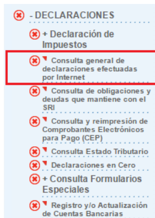
Figura 2.1.2: Menú
